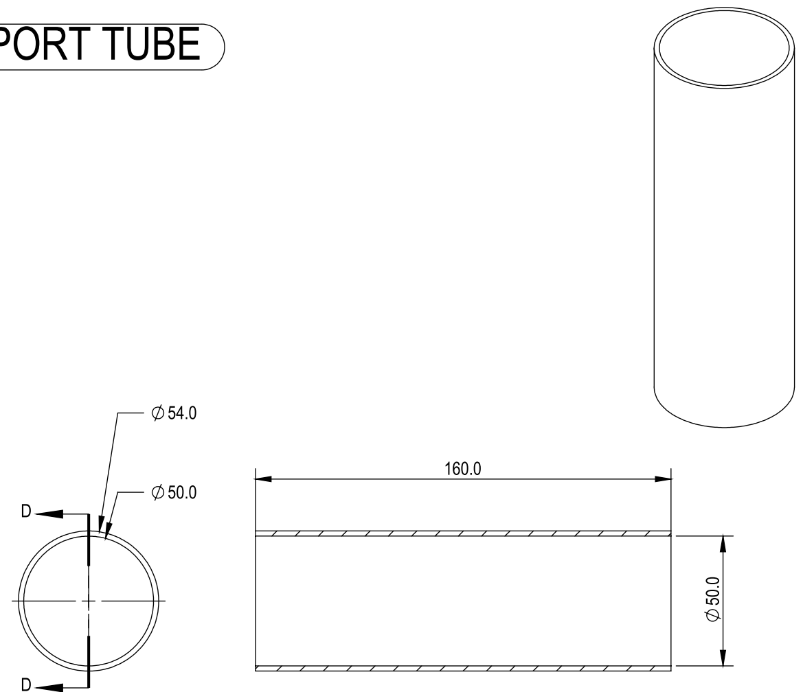
SECTION D-D
